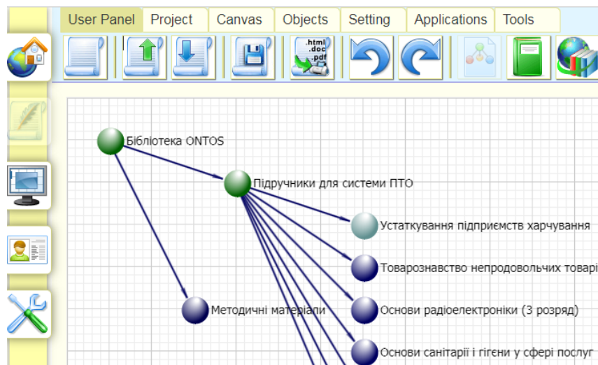
Рис. 1. Вебресурс OntOS
